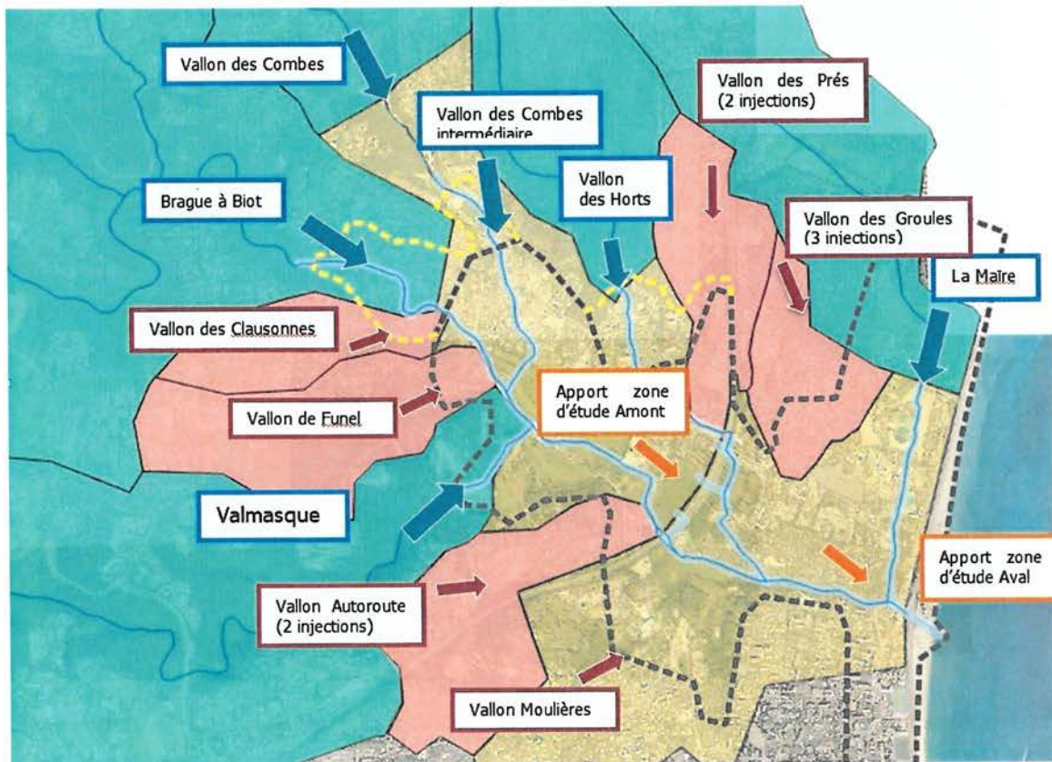
FIGURE 47 : INJECTION DES HYDROGRAMMES DANS LE MODELE 1D/2D
